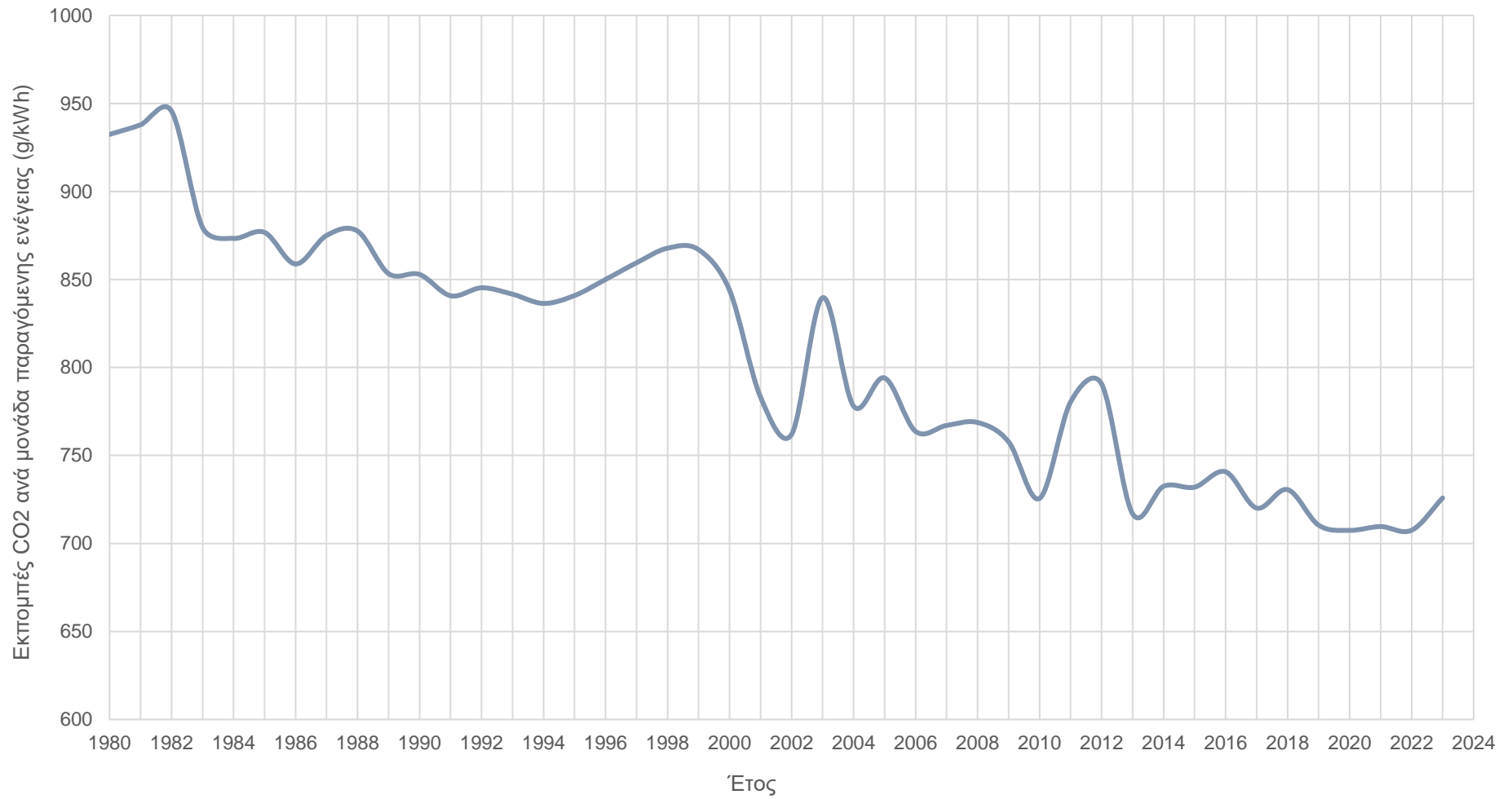
Γράφημα - Ετήσια διακύμανση περιβαλλοντικού δείκτη εκπομπών διοξειδίου του άνθρακα (CO 2 ) σε γραμμάρια ανά κιλοβατώρα από συμβατικές μονάδες ηλεκτροπαραγωγής μεγάλης κλίμακας
